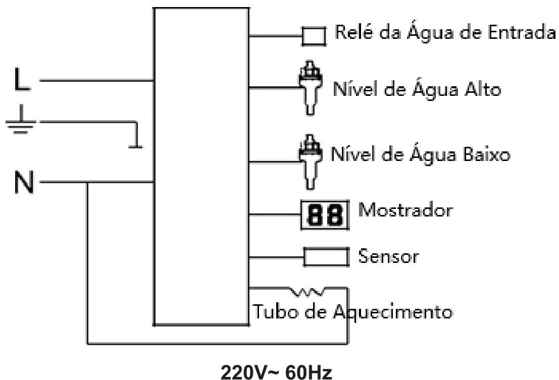
Diagrama do circuito da Caldeira Elétrica de Aquecimento de Água Comercial
